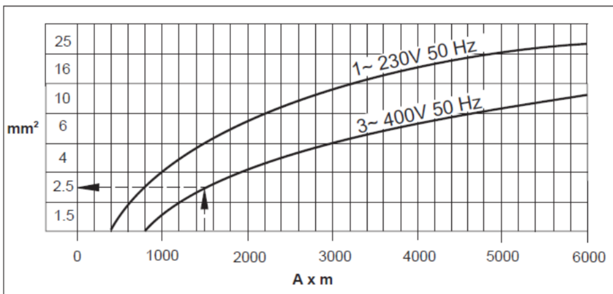
Schemat minimalnego rozmiaru kabla przedłużającego
